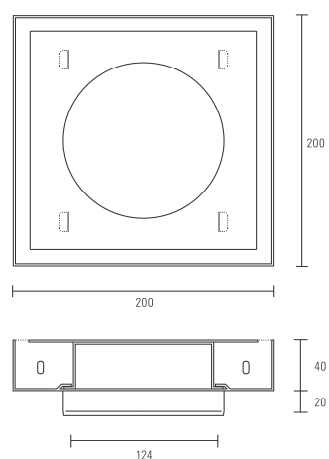
Soupape VAZUM Ø 125 mm
