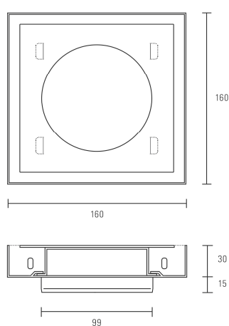
Soupape VAZUM Ø 100 mm
