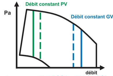
Fonctionnement EXAECO® + MAC2 EC®
