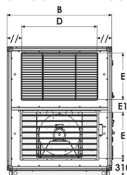
VUE CÔTÉ EXAECO®
