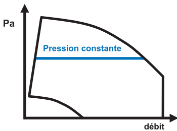
Fonctionnement EXAECO® + LOBBY EC®
